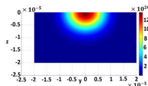
شکل ۲: توزیع عرضی غلظت تیتانیوم در موجبر کانالی با شرایط نفوذ W=10\mu ، \tau=180\text{nm} ، t=17\text{h} ، T=1050^\circ\text{C} .
