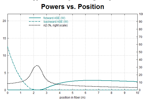
شکل ۵: در غیاب سیگنال و در توان پمپ 20W
