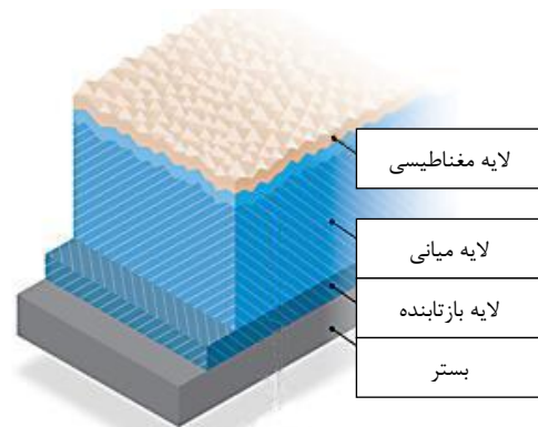
شکل ۱: طرحواره ساختار چندلایه شامل زیرلایه، لایه بازتابنده، لایه میانی و لایه مغناطیسی.
