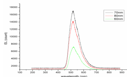
شکل ۳: طیف الکترولومینسانس ساختارهای ۱ و ۲ و ۳
