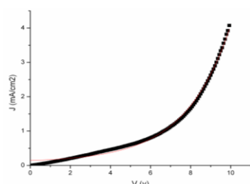
شکل ۲-الف: نمودار ولتاژ-جریان ساختار
