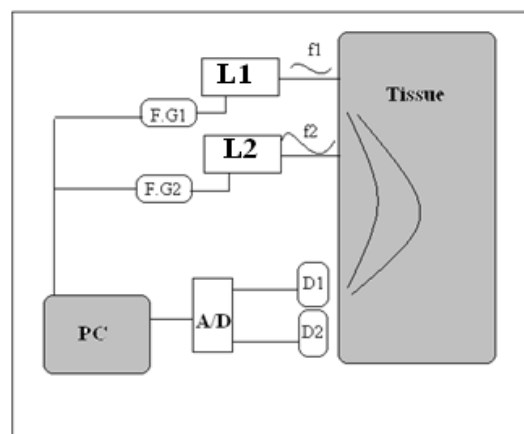
شکل ۱: شماتیکی از سامانه FNIRS که توسط دو لیزر L1 و L2 بافت را نوردهی می‌کند. نور توسط دو آشکارساز D1 و D2 ثبت و اطلاعات به رایانه ارسال می‌شود. F.G.1 و F.G.2 به ترتیب دو فانکشن ژنراتور برای تولید نور مدولاسیون شدتی هستند.
