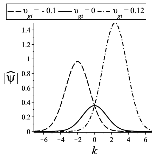
شکل ۱: نمایه پالس گاوسی در فضای پیکربندی و فضای فوریه در t = 10 و برای مقادیر مختلف v_{gi} ( s_i = s_r = 0 ).
