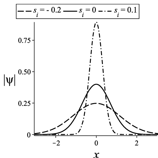
شکل ۲: نمایه پالس گاوسی در فضای پیکربندی در t = 2 و برای مقادیر مختلف s_i ( v_{gi} = s_r = 0 ).
