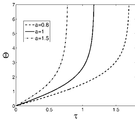
شکل ۲: تحول زمانی جابجایی فاز پرتو گاوسی (چهارچوب بالا) و پرتو سکانت هایپرولیک (چهارچوب پایین).
