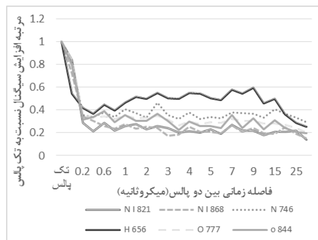
شکل ۴: تأثیر فاصله زمانی دو پالس لیزر بر افزایش شدت تابش پلاسمای برای خطوط طیفی عناصر هوا
