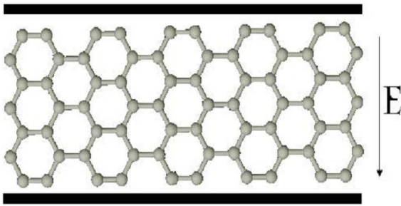
شکل ۱: اعمال میدان در جهت عرضی توسط دو الکترود در لبه بالا و پایینی نانو روبان گرافن. میدان می توان ثابت و یا مدوله شده باشد.
