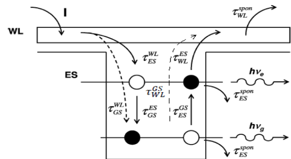
شکل ۱: نمودار طرحواره از مدل واهلش و فرار در لیزر نقطه کوانتومی InAs-InP
