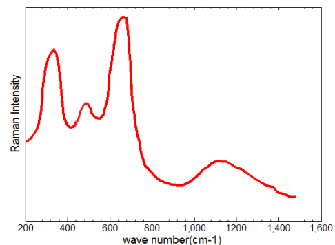
شکل ۳: طیف رامان فریت روی
