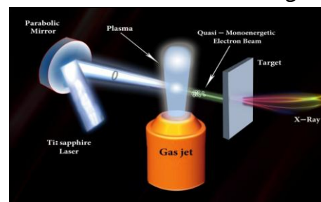
شکل ۱: شمایی از تولید اشعه ایکس، شامل برهمکنش لیزر با هدف گازی، و برخورد الکترون‌های پرنرژی تولید شده با هدف جامد.
