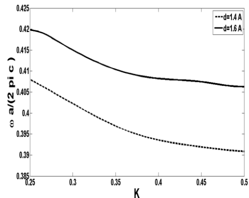
شکل ۷، فرکانس بهنجار بر حسب عدد موج برای مد دوم، دو موجبر با عرض (خط چین) d=1/4A و (خط) d=1/6A
