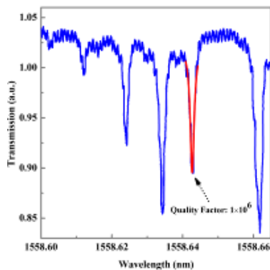
شکل ۵: طیف WGM یک میکروکره با قطر ۴۶۰ \mu\text{m} قطر تیپ ۲ \mu\text{m} حدود است.
