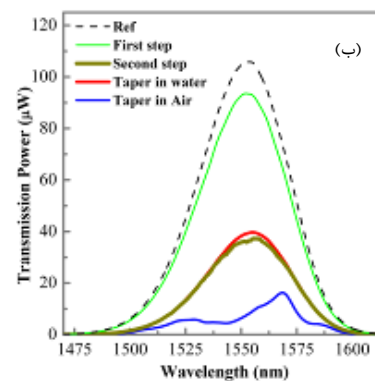
شکل ۴. (الف) طیف عبوری تیپ ساخته شده با قطر نهایی ۱ \mu\text{m} اسید در (P_i)_{\text{max}} \sim P_0/10 خارج شده است (ب) تیپ با قطر نهایی ۲ \mu\text{m} اسید در (P_i)_{\text{max}} \sim P_0/2.5 خارج شده است.
