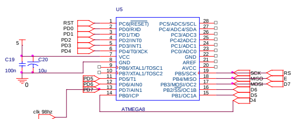
شکل (۶): شماتیک مدار پردازش
