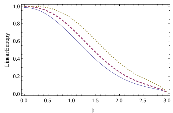
شکل ۲: آنتروپی خطی بر حسب |\alpha| برای تابع پوشل-تالر برای k=3 (خط توپر)، k=4 (خط چین)، k=5 (خط نقطه-خط) و k=6 (خط نقطه).
