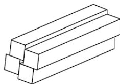
شکل ۲: نمای یک هدایتگر بازتابی متشکل از چهار آینه متصل به یکدیگر
