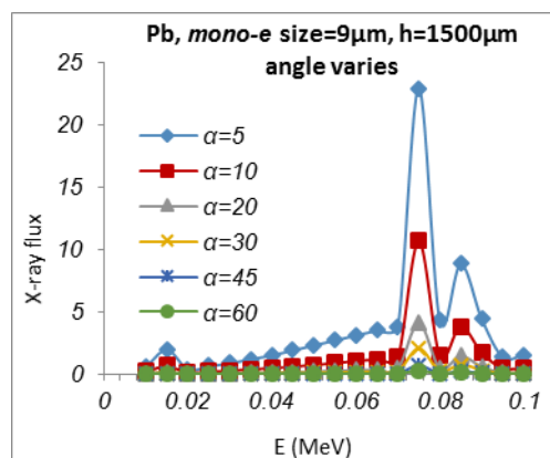
شکل ۱ ب مقایسه هدف مخروطی شکل با زاویه راس های مختلف در ارتفاع 1500\text{ }\mu\text{m} میکرومتر
