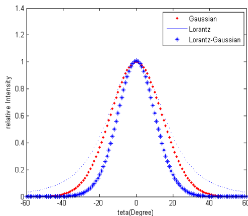
شکل ۱: توزیع شدت میدان گاوسی، لورنتس و لورنتس-گاوسی
