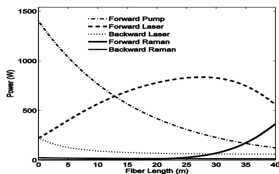
شکل ۱ (ج): رشد موج رامن و کاهش موج لیزر برای دمش از
