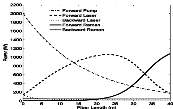
شکل ۱ (د): رشد موج رامن و کاهش موج لیزر برای دمش از
