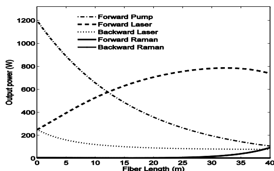
شکل ۱ (الف): رشد موج رامن و کاهش موج لیزر برای دمش از
