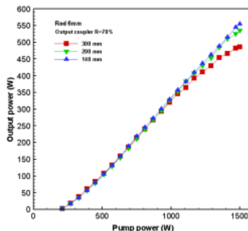
شکل ۵ : توان خروجی برای رزوناتور با آینه‌های تخت، و آینه خروجی ۷۰٪ با طول رزوناتور ۱۴۰ mm، ۲۰۰ mm، ۳۰۰ mm (a) میله لیزری با قطر ۵ mm (b) میله لیزری با قطر ۶ mm
