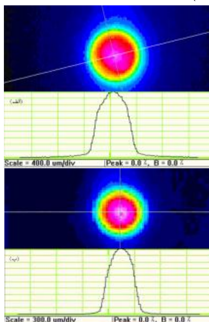
شکل ۴: توزیع فلورسانس اندازه‌گیری شده برای میله لیزری با قطر (الف) 5\text{ mm} (ب) 6\text{ mm} .
