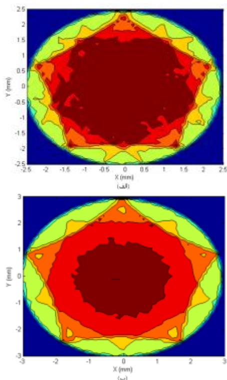
شکل ۳: توزیع توان دمش محاسبه‌شده برای میله لیزری با قطر (الف) 5\text{ mm} (ب) 6\text{ mm} .
