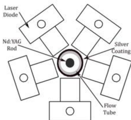
شکل ۱: شمای سامانه دمش جانبی با 5 لیزر دیود به عنوان واحد-های دمش.
