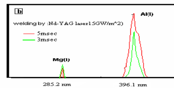
شکل ۳. دو خط مشخصه تابشی، برای دو فلز جوش در پهنای پالسی متفاوت ۳ و ۵msec و چگالی توان تابشی ۱۵GW/m²
