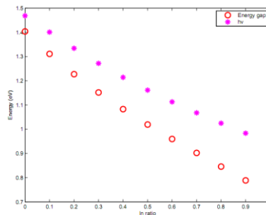
شکل ۷. انرژی بازترکیب الکترون-حفره و گاف نوار بر حسب تغییرات x .
