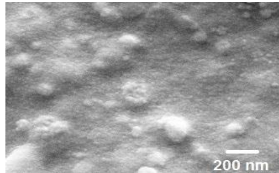
شکل ۳. تصویر گرفته شده توسط FE-SEM از سطح لایه نازک مربوط به نمونه قبل از سینترینگ.
