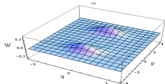
شکل (۱): تابع ویگنر وابسته به زمان در فضای فاز برای حالت‌های همدوس زوج فوتون-افزوده به ازای m = 1, \alpha = 2i با \gamma t = 0.01 : ب، \gamma t = 0.06 و \gamma t = 0.15 .
