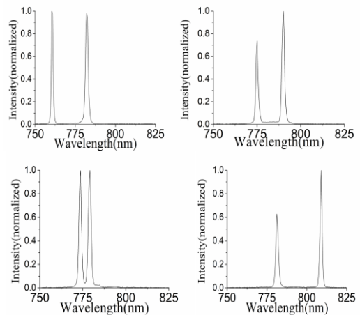
شکل ۲: طیف‌های دو طول موجی خروجی از لیزر کوک‌پذیر دو طول موجی که با چرخش آینه‌های ۱۴ و ۱۵ در زمان‌های مختلف توسط Ocean optics ثبت شده‌اند.
