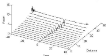
شکل ۳: انتشار سالیتون هنگامی که \tau_R = 0.025 ، \beta = 0.025 ، \delta = 0.0025 و \varepsilon = 0.01475 و \mu = 0
