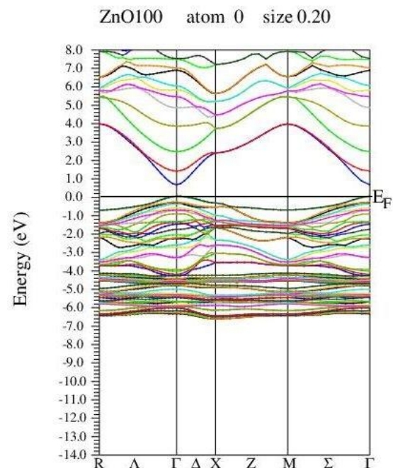
شکل ۴: ساختار نواری فیلم نازک رشد داده شده در راستای [10-10]
