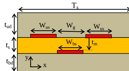
شکل ۱: هندسه‌ی یک موجبر شبه مسطح QCPW.
