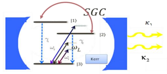
شکل ۱: طرحواره از اتم سه تراز با همراه با غیرخطیت کر درون کاواک دو مدی.
