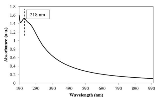
شکل ۲: طیف جذب مرئی-فراپیش حاصل از سنتز لیزری نانوذرات پلاتین در محیط آب مقطر.
