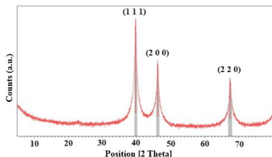
شکل ۳: طیف پراش اشعه ایکس که از پودر حاصل از نانوذرات پلاتین گرفته شده است.
