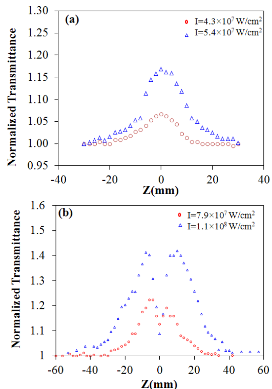
شکل ۴: نتایج حاصل از تابشدهی نانوذرات پلاتین با شدت‌های تابشی مختلف در آزمایش روزنه باز روبش Z
