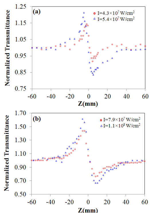
شکل ۵: نتایج حاصل از تابشدهی نانوذرات پلاتین با شدت‌های تابشی مختلف در آزمایش روزنه بسته روبش Z
