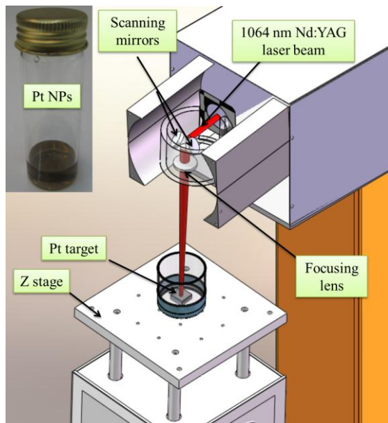
شکل ۱: چیدمان آزمایشگاهی برای سنتز نانوذرات پلاتین به روش کند و سوز لیزری در محیط آب مقطر
