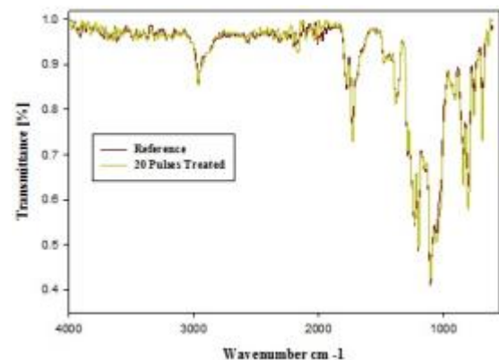
شکل ۳. طیف نشری FTIR لنز قبل و پس از پرتو دهی با
