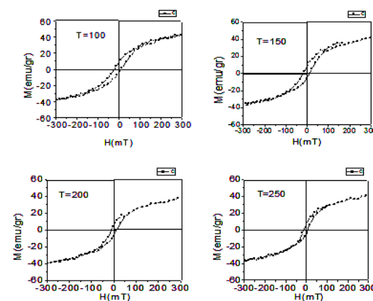
شکل ۳- منحنی پسماند نمونه ۳ در دماهای مختلف
