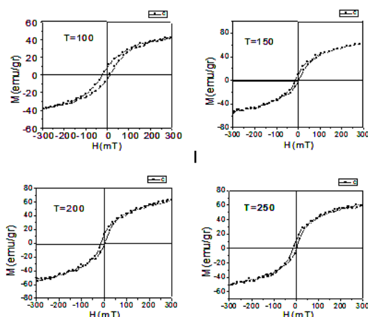
شکل ۲- منحنی پسماند برای نمونه ۲ در دماهای مختلف
