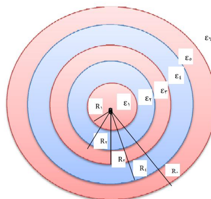
شکل (۱) سطح مقطع نانوشل کروی یا استوانه ای ۵ لایه
