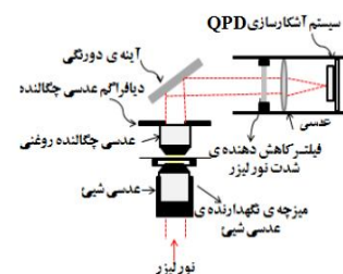
شکل ۱- چیدمان مورد استفاده در آزمایش.
