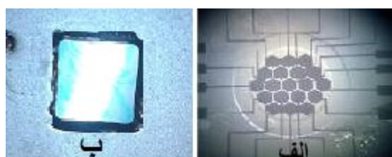
شکل ۳: (الف) تصویری از الکتروودهای شش ضلعی به همراه دیواره (ب) دیافراگم پلیمری
