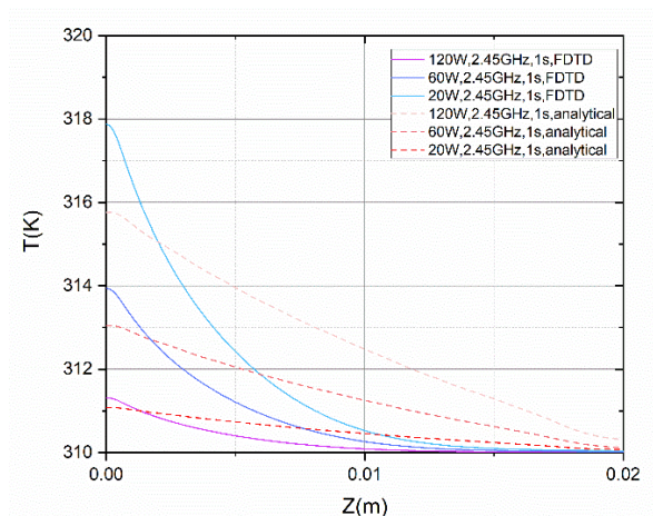
شکل ۳: مقایسه حل تحلیلی و عددی برای توان های مختلف در فرکانس ۲.۴ گیگاهرتز. در نمودار، خطوط پیوسته جواب عددی و خطوط گسسته پاسخ تحلیلی را نشان می دهند.
