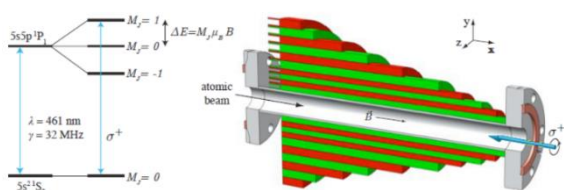
شکل ۱: کند کننده زمین. پرتو لیزر با طول موج ۴۶۱ نانومتر ویلازیاسیون مثبت اتمهای خارج شده از کوره را کند می کند.
