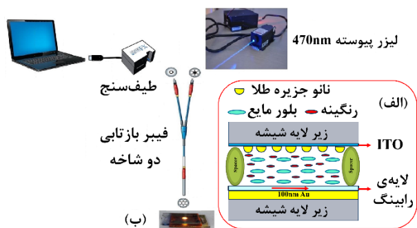
شکل ۱: شماتیک مربوط به (الف) کاواک فابری پرو حاوی بلور مایع و رنگینه، (ب) چیدمان آزمایش طیف فلوئورسانس.
