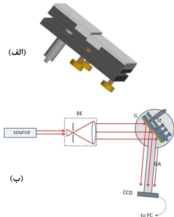
شکل ۳: (الف) طرح پله استفاده شده در آزمایش. (ب) چیدمان آزمایش. BE باریکه گستر، G گونیومتر، GA بازوی گونیومتر، St پله
