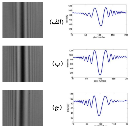
شکل ۲: نقش‌های پراش و نمایه های شدت آنها برای نور پراشیده از پله وقتی که اختلاف فاز الف) \varphi = (2m+1/2)\pi ، ب) \varphi = (2m+3/2)\pi ج) \varphi = (2m+1)\pi است. عدد صحیح m است.
