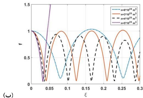
شکل ۱: تغییرات شعاع لکه لیزری برای چگالی الکترونی با الف) پروفایل نمایی و ب) پروفایل خطی برای حالتی که \alpha_0 A_0^2 = 0.3
