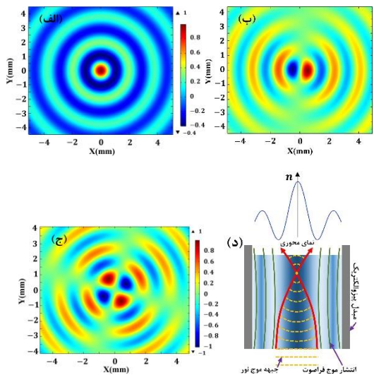
شکل ۳: الگوهای تداخل فضاوی تولید شده در فانتوم بافت مغز توسط موج فشاری فراصوت. به ازای ولتاژ ورودی ۳۴ v (الف) مد پایه ( m = 0 ) در فرکانس ۸۲۸،۶۴ kHz (ب) مد مرتبه دوم ( m = 1 ) در فرکانس ۸۴۸،۰۵ kHz (ج) مد مرتبه سوم ( m = 2 ) در فرکانس ۸۶۷،۲۸ kHz (د) شماتیک مدولاسیون ضریب شکست و هدایت نور درون فانتوم با تشکیل امواج ایستاده فراصوت.
