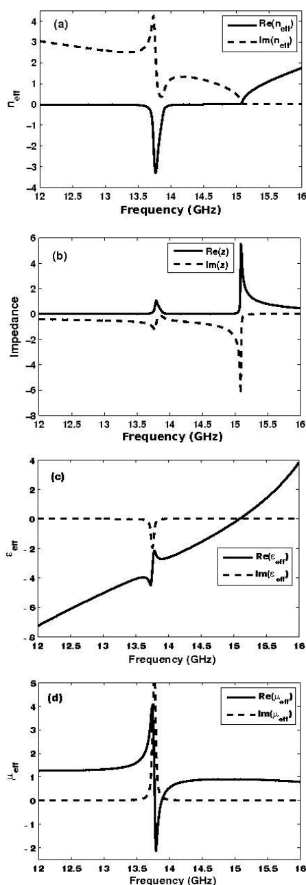
شکل ۳: مقادیر محاسبه شده ی ضریب شکست (a)، امپدانس (b)، ضریب گذردی الکتریکی (c) و تراوایی نسبی مغناطیسی (d) برای ساختار نشان داده شده در شکل ۱.
