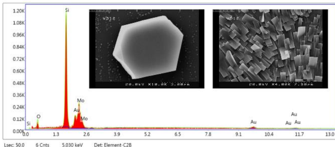
شکل ۳: تصاویر میکروسکوپ روبشی و edx از ورقه های \text{MoS}_2
