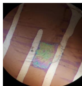
شکل ۴: تصویر میکروسکوپ لایه \text{MoS}_2 بین الکترودهای نیکل
