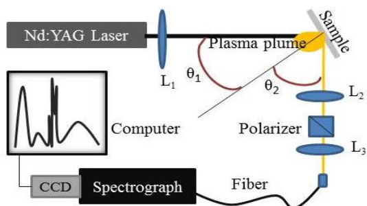
شکل ۱. طرحواره‌ای از چیدمان آزمایش.
