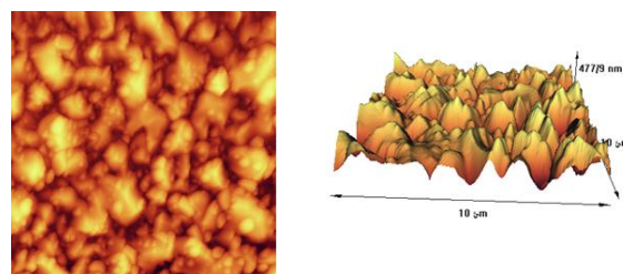
شکل ۵: تصاویر AFM برای لایه نازک نوعی \text{TeO}_2
