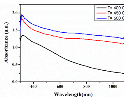
شکل ۶: طیف جذب لایه‌های نازک \text{TeO}_2 تهیه شده در دماهای ۴۰۰ °C، ۴۵۰ °C و ۵۰۰ °C
