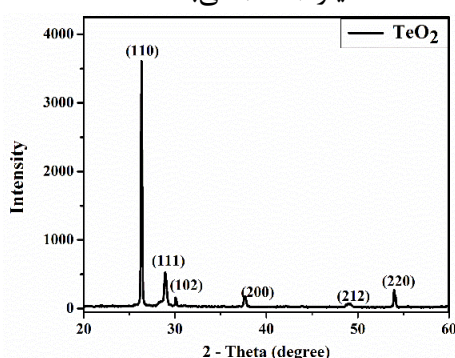
شکل ۱: طیف XRD برای لایه نازک \text{TeO}_2
