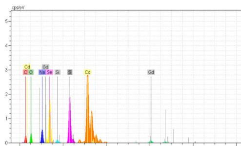
شکل ۲: طیف پراش انرژی اشعه ایکس نقاط کوانتوم آلاینده به گادولینیوم
