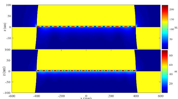
شکل ۴: توزیع میدان الکتریکی در ساختار پیشنهادی. شکل بالایی توزیع میدان در فرکانس ۴۱ تراهرتز است که دارای مرتبه‌ی رزونانس ۱۱ است و متناظر با پیک نور بازگشتی است. شکل پایینی توزیع میدان در فرکانس ۴۸/۲۳ تراهرتز است که دارای مرتبه‌ی رزونانس ۱۸ بوده و متناظر با دره‌ی طیف نور بازگشتی است
